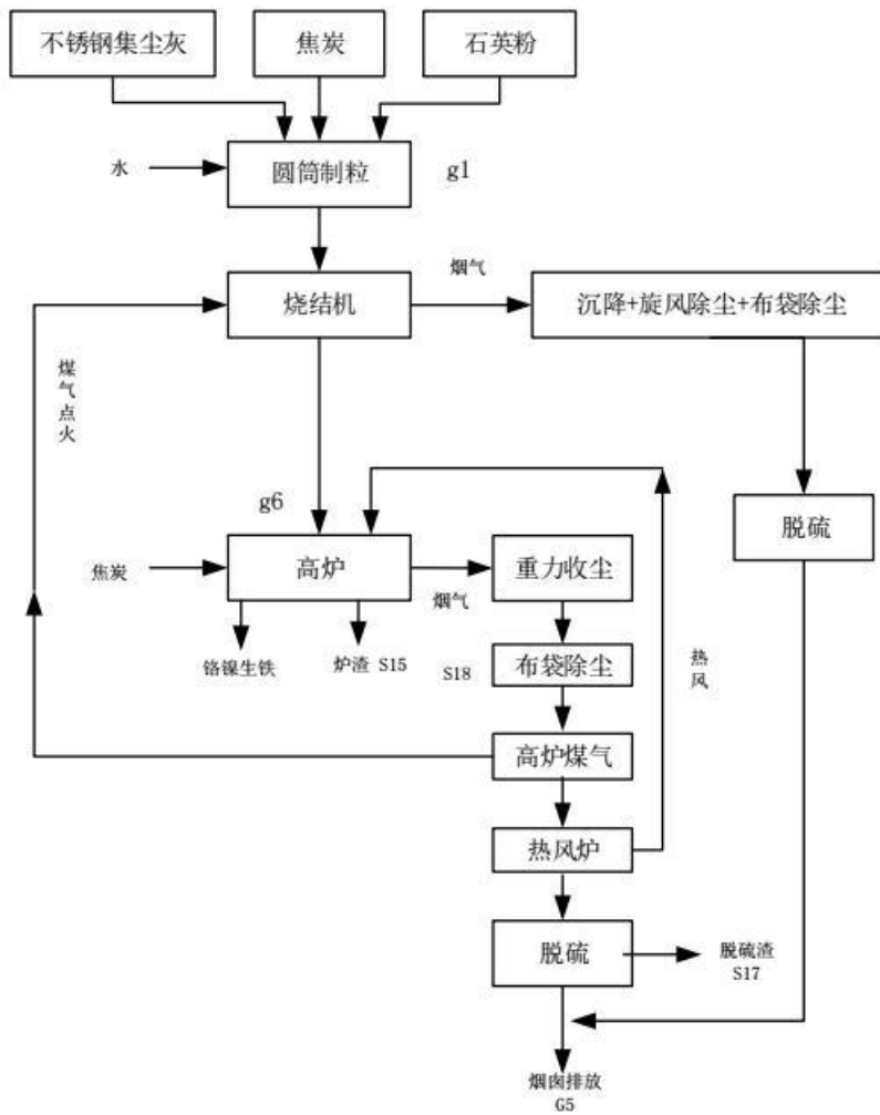
图 2.4-3 不锈钢除尘灰综合利用工艺流程图
