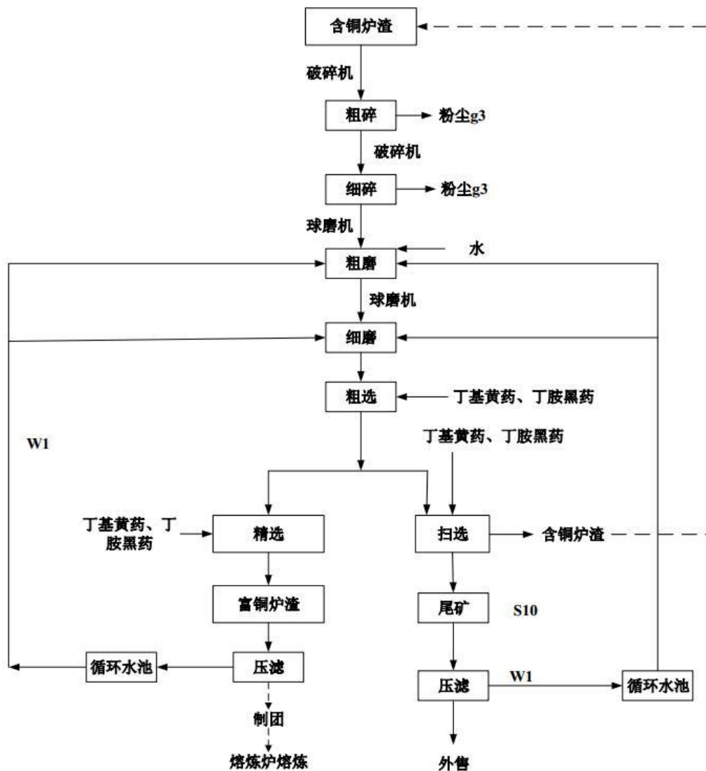
图 2.4-4 含铜炉渣浮选工艺流程图
