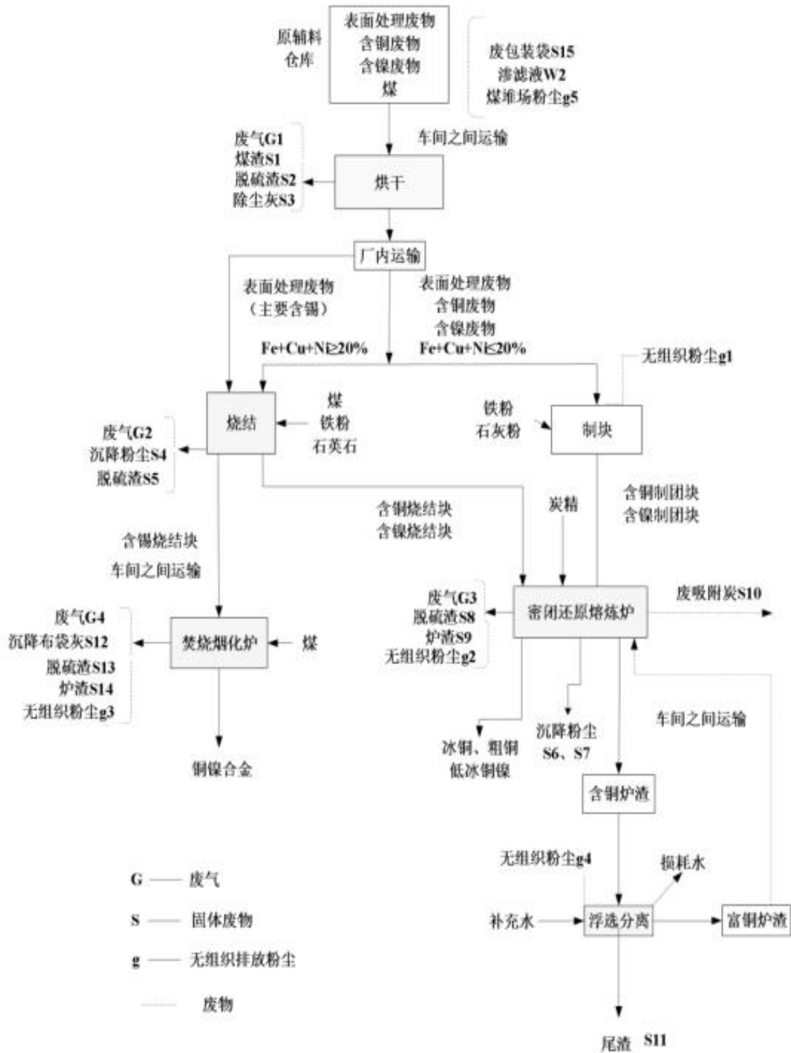
图 2.4-1 主要生产工艺流程及产污环节简图
